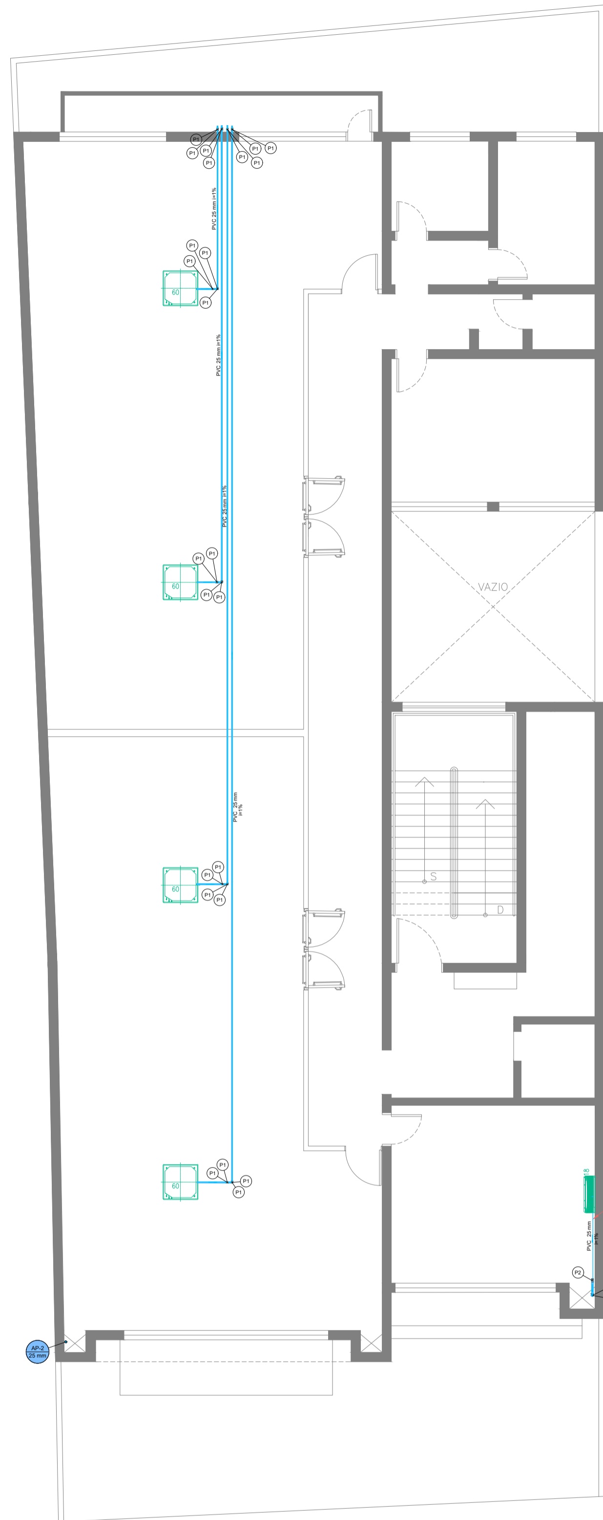
Planta baixa 3º Pavimento Escala 1:100
